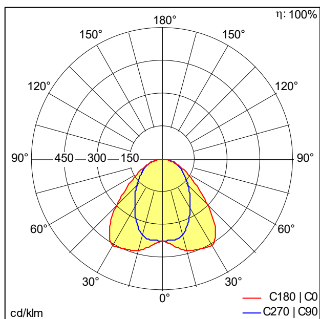
TECTON_C_5500_830_L1500_VWB_LDE_WH.Idt
