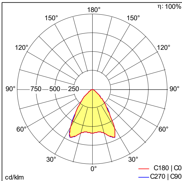
D43023_MIRL_LAY_3800-840_M625L_NB_LDO_WH.Idt
