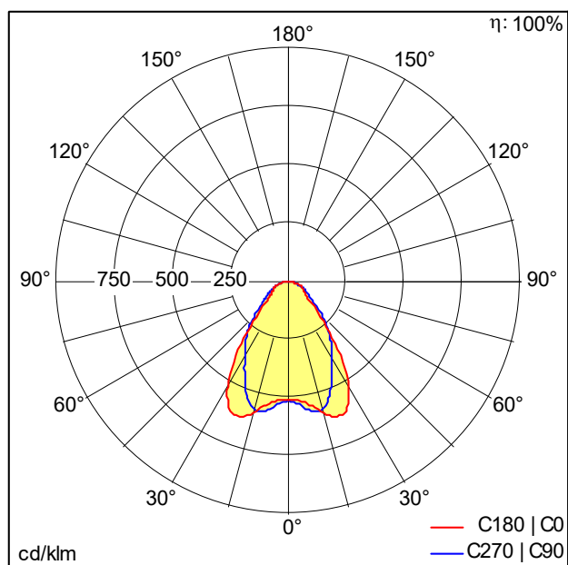
D35001_TECTON_C_8000-865_L1500_WB_LDE_WH.Idt
