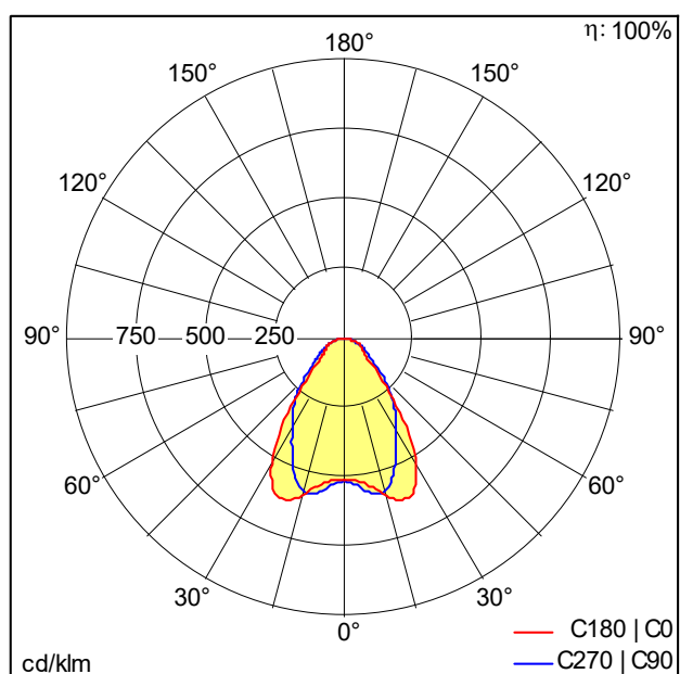
D35001_TECTON_C_5500-840_L1500_WB_LDE_SR.Idt
