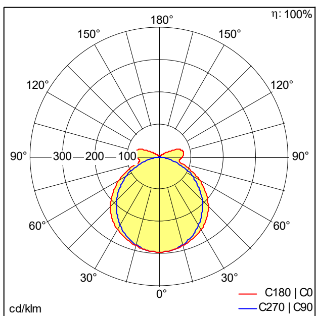
D45908_AMP_L_BAS_4600-840_PC_MB_LDO.idt
