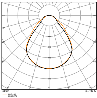
PL COMP 625 DA V 30W 930 U19 4200lm
