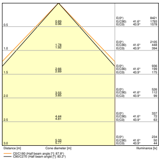
PL COMP 625 DA V 30W 940 U19 4200lm
