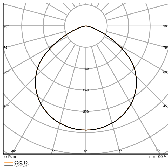
FL COMP 30 50 42W 840 100 WT
