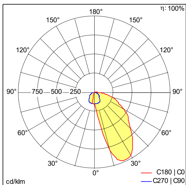
D34983_TECTON_C_5500-830_L1500_WW_LDE_WH.Idt
