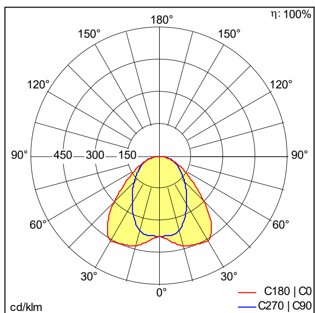
TECTON_C_5500_840_L1500_VWB_LDE_WH.Idt
