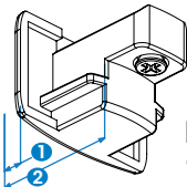
End cap GB 41 1. 4 mm, 2. 24 mm
