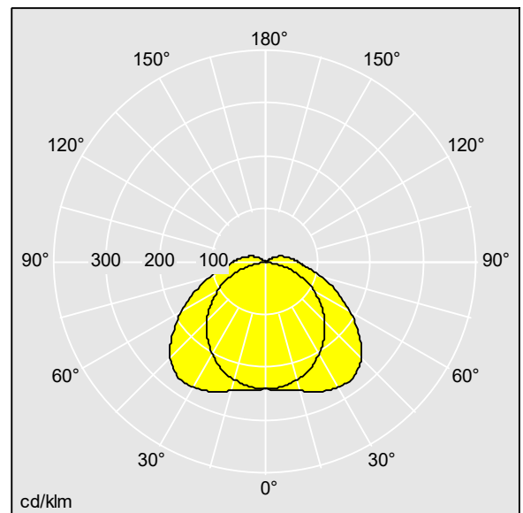
D45932_AQFPRO_L_10000-840_PC_WB_HF.ltd
