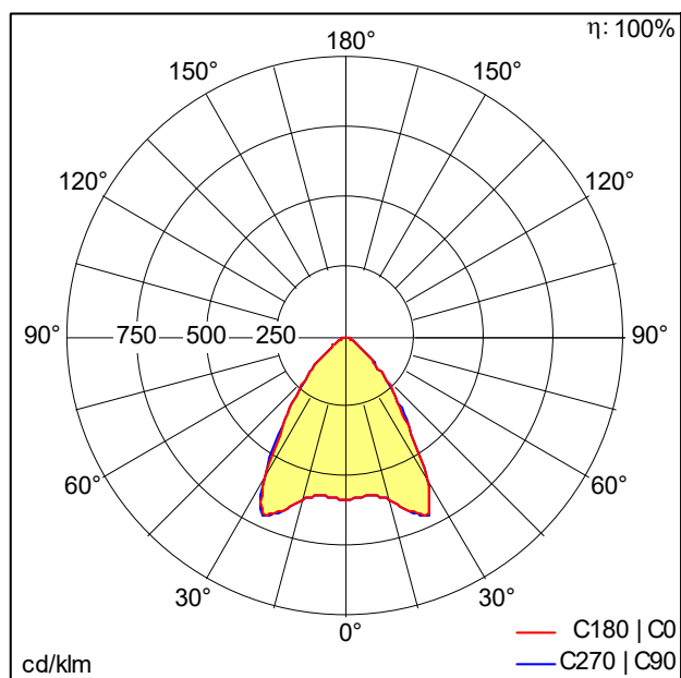
D43023 MIRL NIV 3800-840 M625L NB LDO WH.Idt
