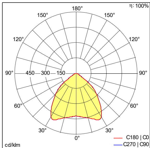
D43022_MIRL_LAY_3800-840_M625Q_WB_LDO_WH.Idt
