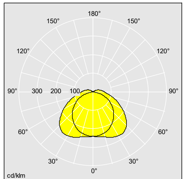
D45932_AQFPRO_L_4300-840_PC_WB_HF.Idt
