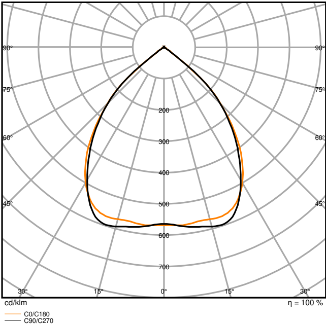
PL INV 625 ZB P 38W 940 U19 BK-800mA
