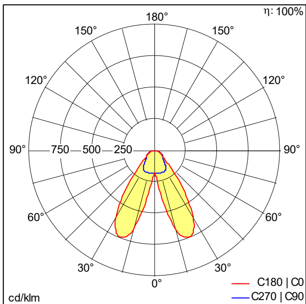
D43655_TECTON_C_5200-830_L1000_SB_LDE_WH.Idt
