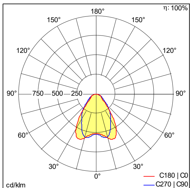
D35001_TECTON_C_12000-865_L1500_WB_LDE_WH.Idt
