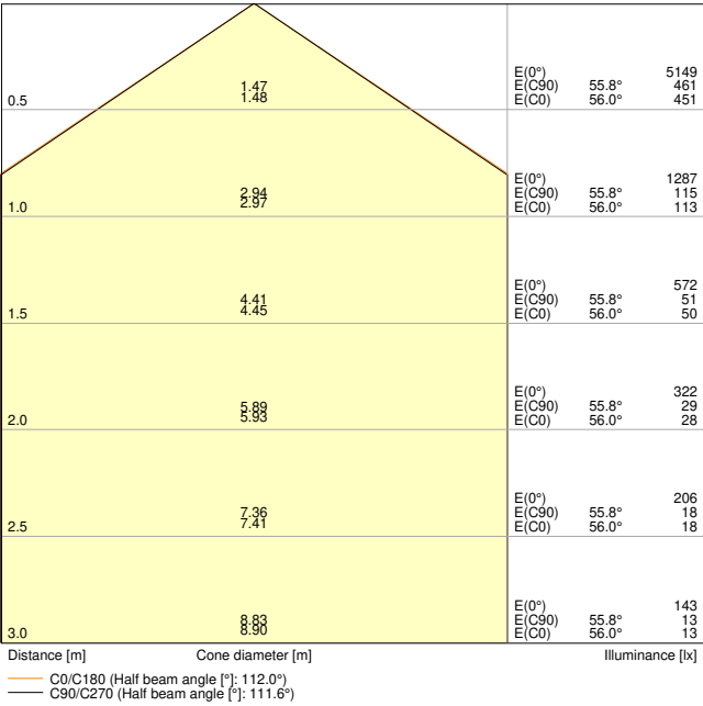
PL COMP 625 V 26W 840 3640lm
